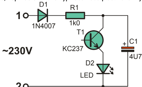
Obr. 1. schéma zapojení
